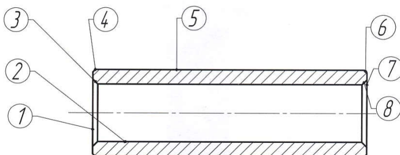
Рис. 1 Эскиз пальца поршневого
